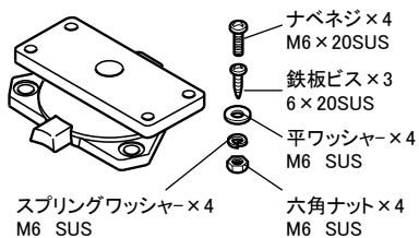
ロータリー架台 (RK05)
