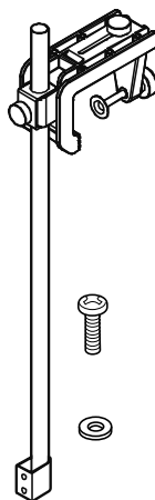
万能パイプ取付金具 (BP10)
