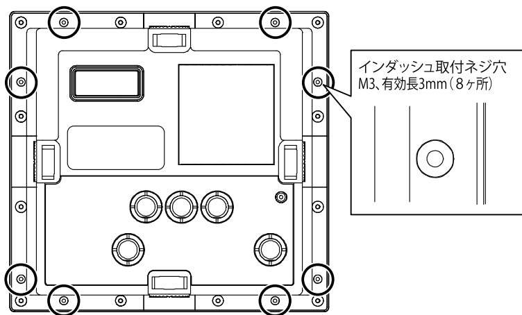
本体裏側
