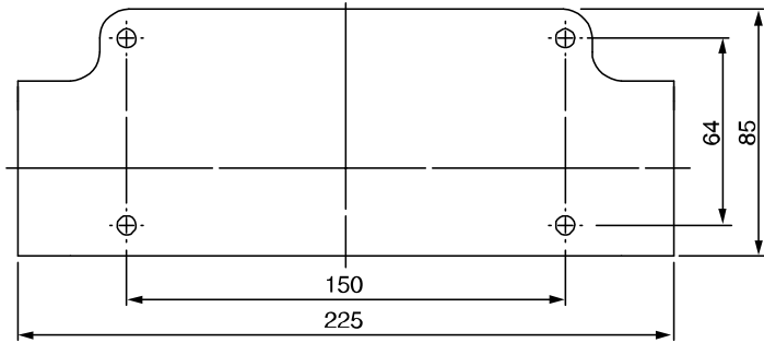
〈架台取付け穴寸法図〉
