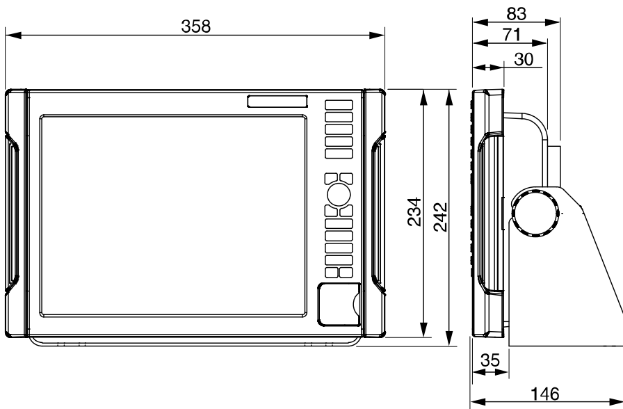
<本体寸法図>
